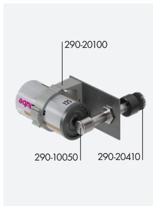
Pinceau avec pièce de raccordement à 90°
