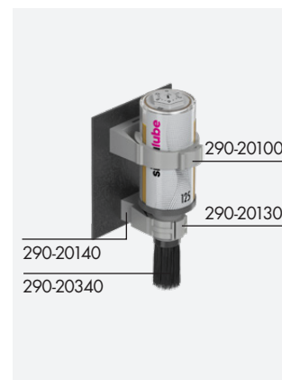
Lubricación de cadena con pincel y dos abrazaderas
