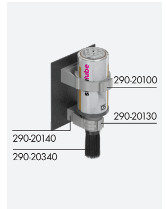
Kettenschmierung mit Pinsel und 2 Halteschellen
