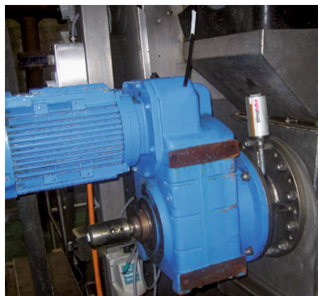
Lubrificazione dell'albero principale di una pressa di lavaggio.
