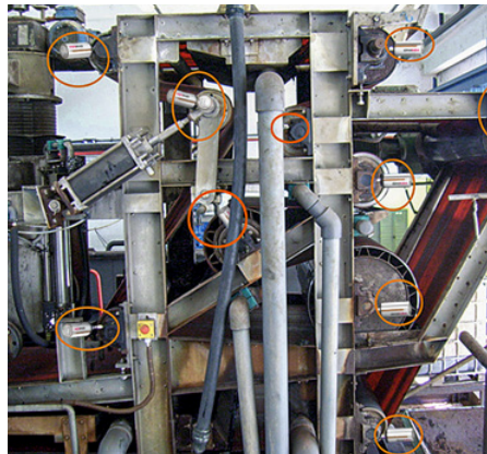
Filtro pressa a nastro con numerosi punti di lubrificazione trattati con simalube.
