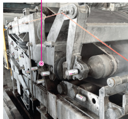
Diversi simalube 125 ml lubrificano i cuscinetti di una macchina per la carta in modo automatico e preciso.
